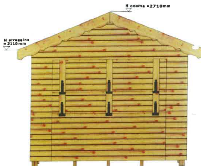
Schița tehnică a căsuței și imagini cu aceasta montată Model decorare căsuță
