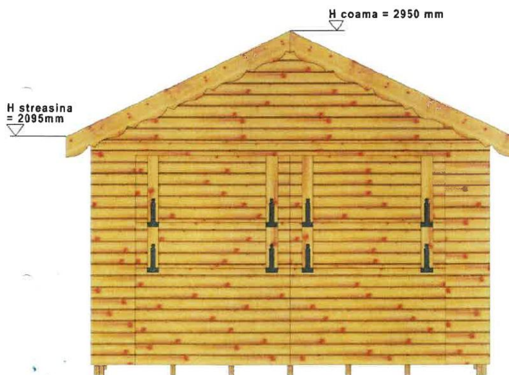
Schița tehnică a căsuței
